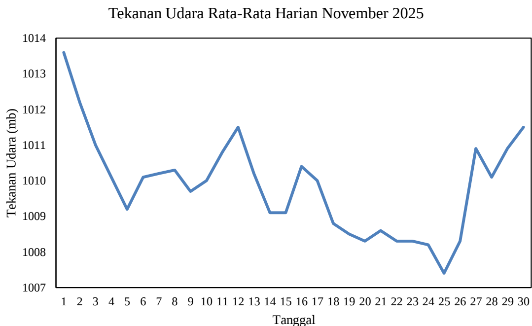
Gambar 2.6 Grafik Tekanan Udara Rata-rata Harian bulan November 2025 di Stasiun Meteorologi Mali - Alor
