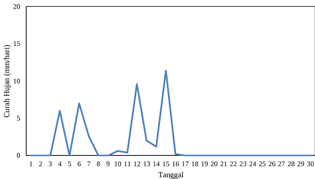
Gambar 2.4 Grafik Curah Hujan Harian November 2025 di Stasiun Meteorologi Mali - Alor
