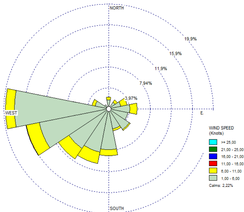
Gambar 2.9 Wind Rose Angin Permukaan Bulan November 2025 di Stasiun Meteorologi Mali - Alor
