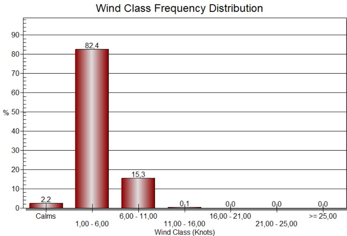
Gambar 2.10 Distribusi Frekuensi Angin Permukaan Bulan November 2025 di Stasiun Meteorologi Mali - Alor
