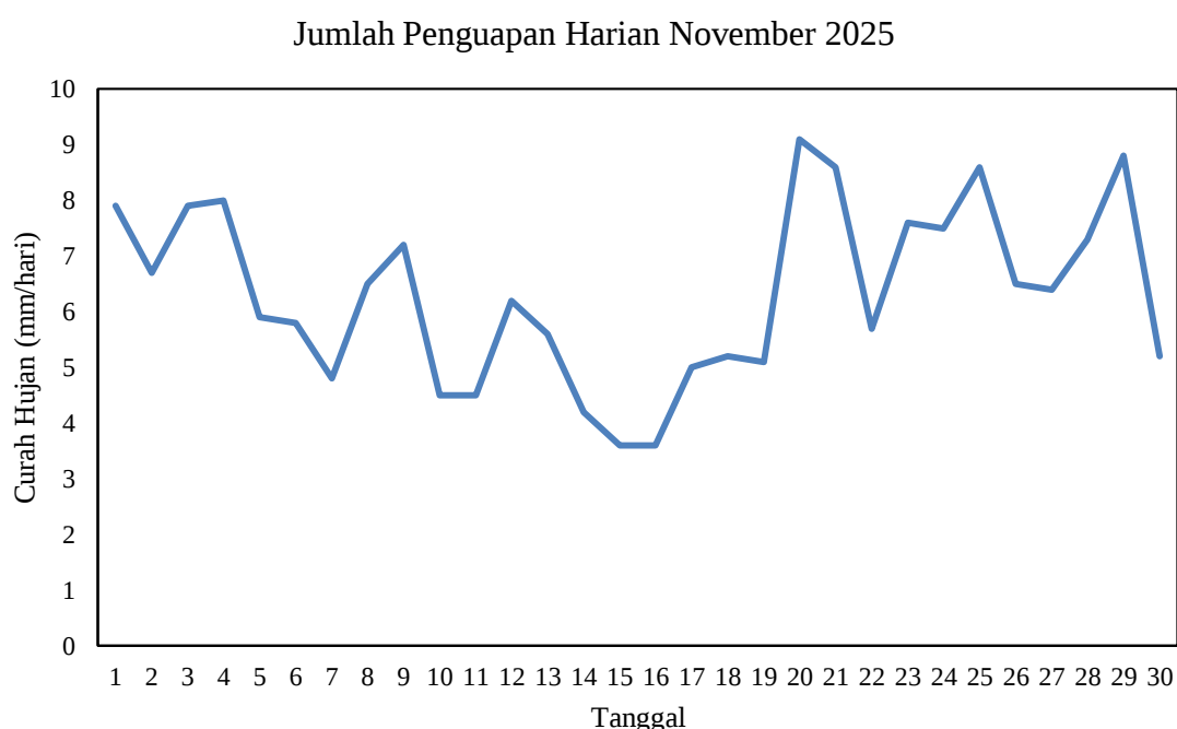
Gambar 2.8 Grafik Jumlah Penguapan Harian bulan November 2025 di Stasiun Meteorologi Mali - Alor
