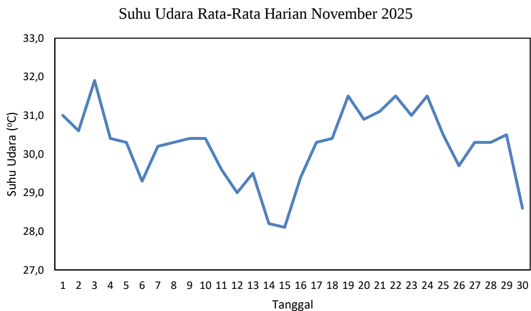
Gambar 2.1 Grafik Suhu Udara Rata-rata Harian Bulan November 2025 di Stasiun Meteorologi Mali - Alor
