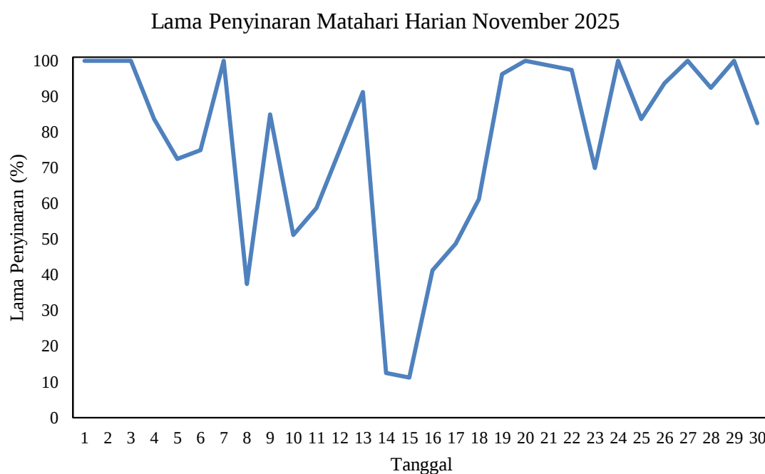
Gambar 2.7 Grafik Lama Penyinaran Matahari Harian bulan November 2025 di Stasiun Meteorologi Mali - Alor
