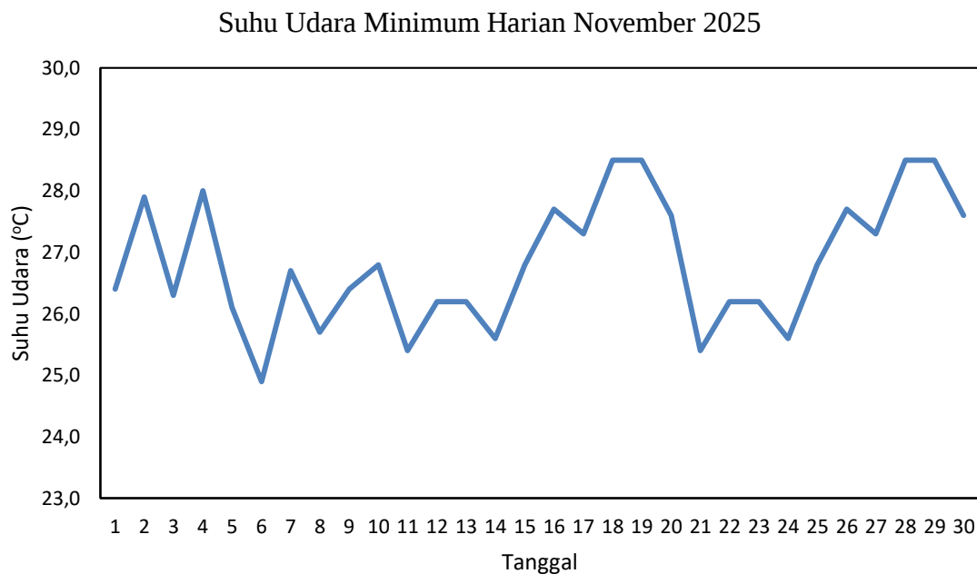
c Gambar 2.3 Grafik Suhu Udara Minimum November 2025 di Stasiun Meteorologi Mali - Alor
