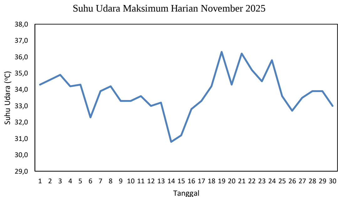
Gambar 2.2 Grafik Suhu Udara Maksimum November 2025 di Stasiun Meteorologi Mali - Alor
